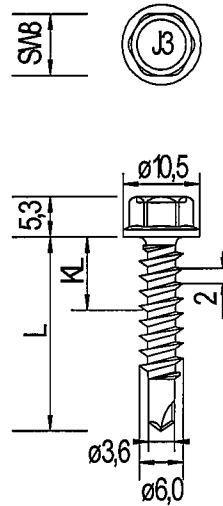
Bohrschraube JT3-2-6,0 x L
