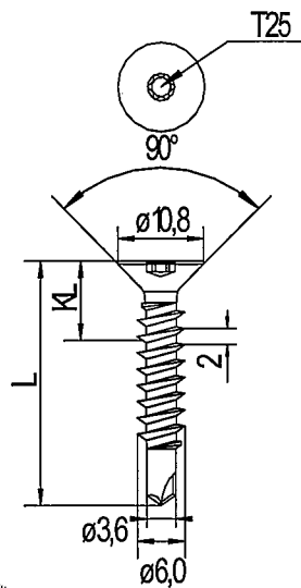
Bohrschraube JT3-ST-2-6,0 x L Bohrschraube JT2-ST-2-6,0 x L
