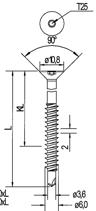
Bohrschraube JT3-ST-2-6,0 x L Bohrschraube JT2-ST-2-6,0 x L
