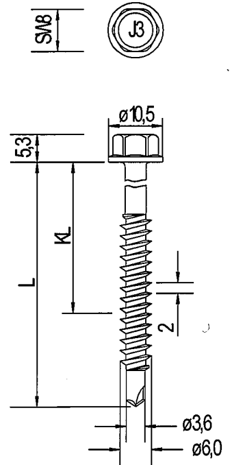
Bohrschraube JT3-2-6,0 x L
