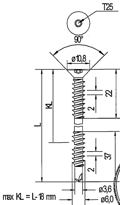
Bohrschraube JT3-ST-2-6,0 x L / UG
